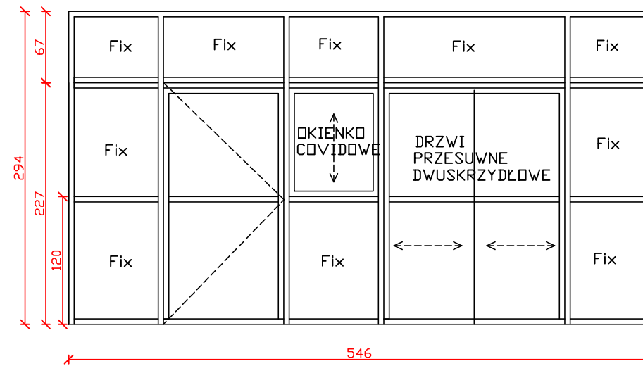
WIDOK OD ZEWNĄTRZ 1:50
