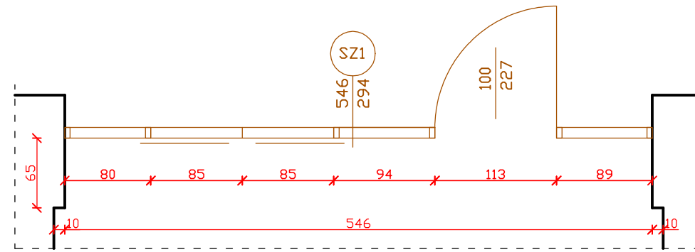
RZUT PRZYZIEMIA 1:50
